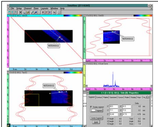
Obr. 7 - Analýza údajov v 2-D zobrazení na referenčnom bloku. Referenčné chyby sú zárezy 6 mm x 2 mm v žľabe č.3.
